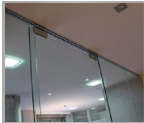
Guía enrasada a techo.
